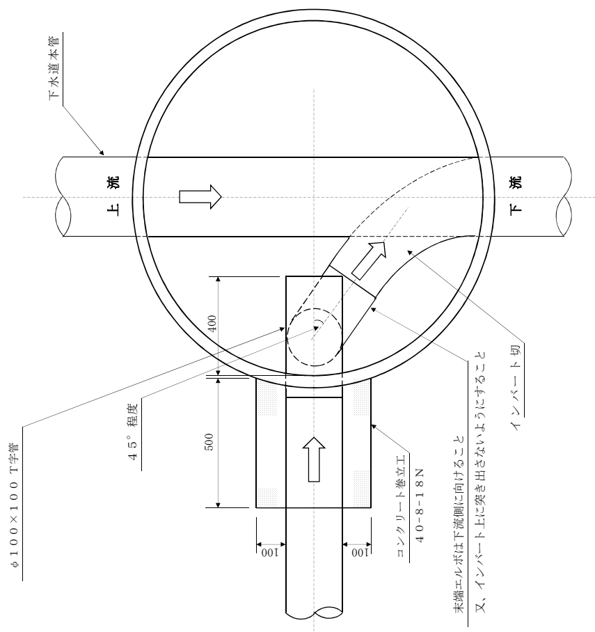
インバート部平面図
