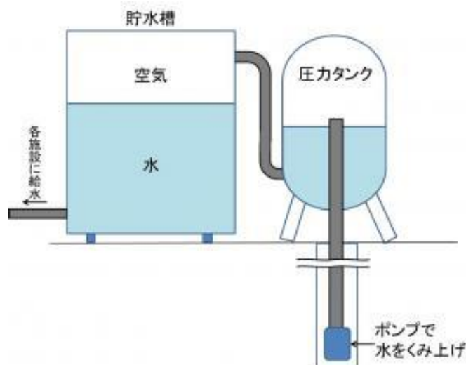
小規模水道施設の圧カタンク 概略図
